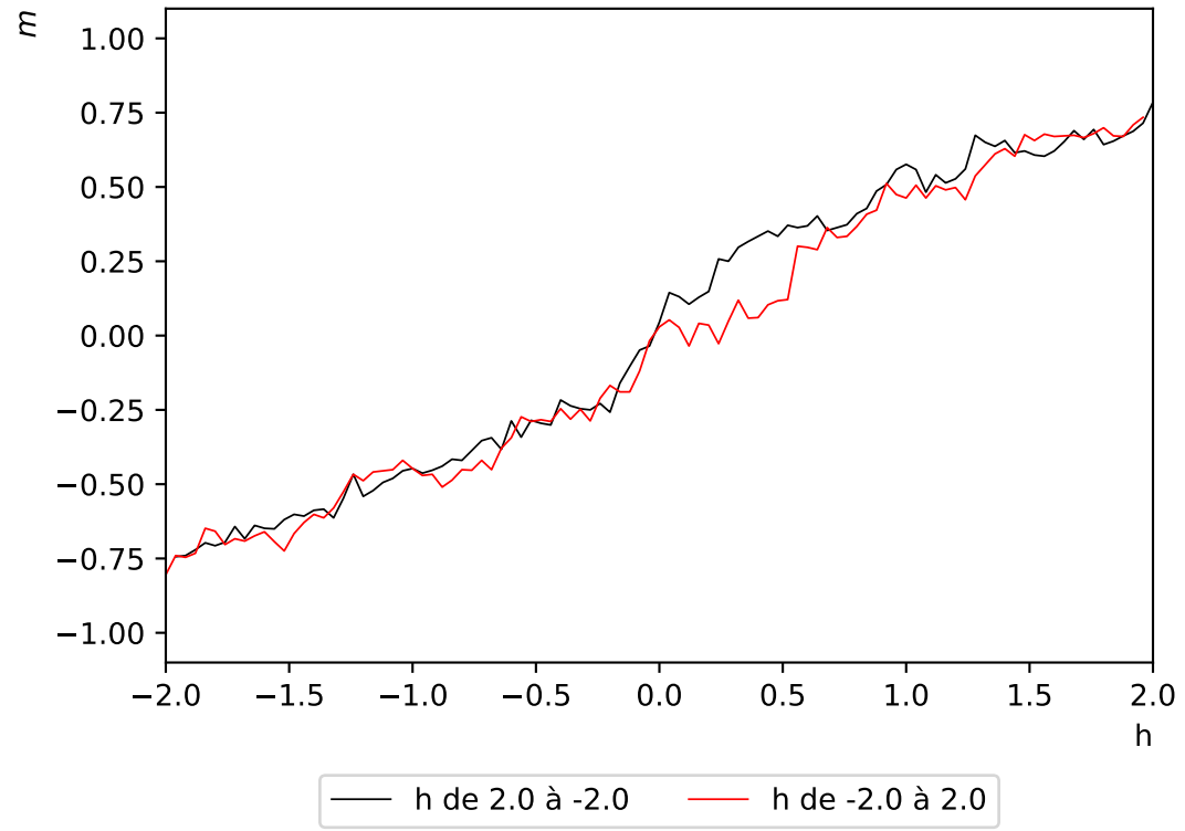
Hystérésis de l'aimantation - réseau de taille L=32 - champ magnétique d'amplitude h=2 à T=5.0
